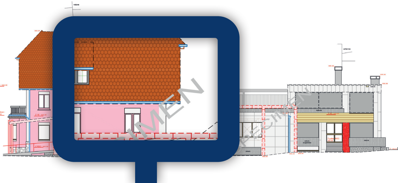
EXEMPLE DE PLANS DE FAÇADE ET DE COUPE D'UN BÂTIMENT PATRIMONIALE RÉALISÉ À PARTIR D'UN SCAN 3D
